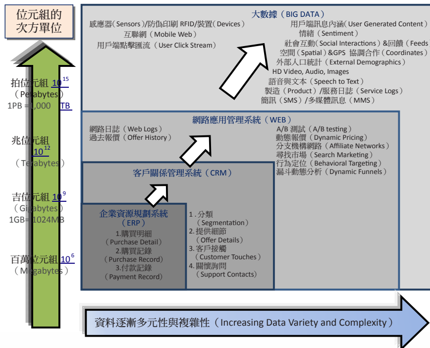
圖 3 大數據示意圖 (資料來源: Contents of created in partnership with Teradata, Inc.)
