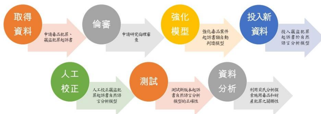
圖 3-2-1 研究流程圖
