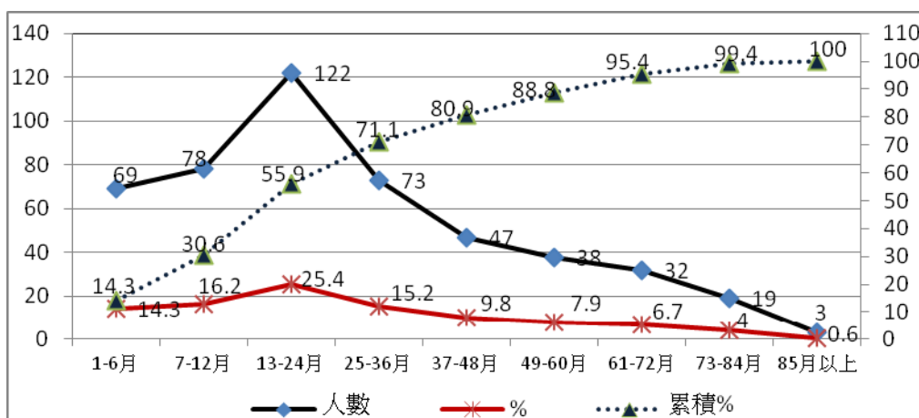
圖 1 再犯組樣本再犯時距分布圖
